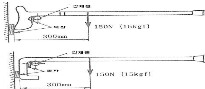
<그림 3> 손잡이 굽힘시험
