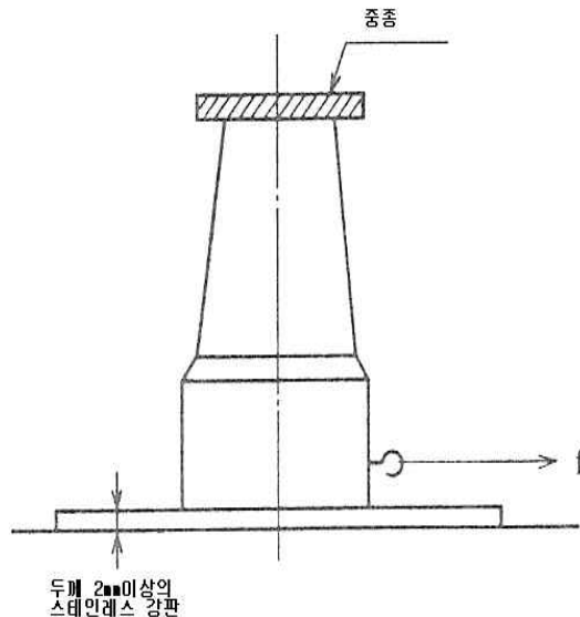
<그림 6> 마찰저항시험
