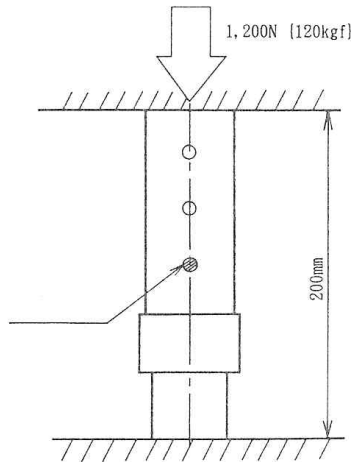
<그림 5> 압축하중시험(조절식지팡이시험 예)
